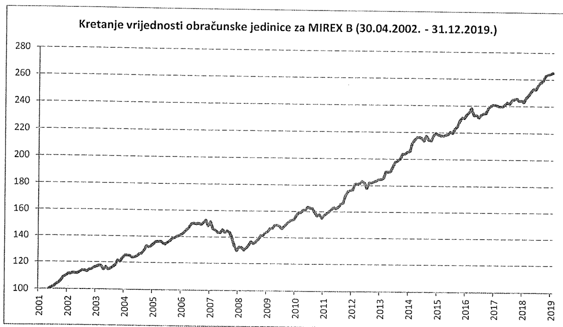
Slika 5: Kretanje vrijednosti indeksa MIREX B
