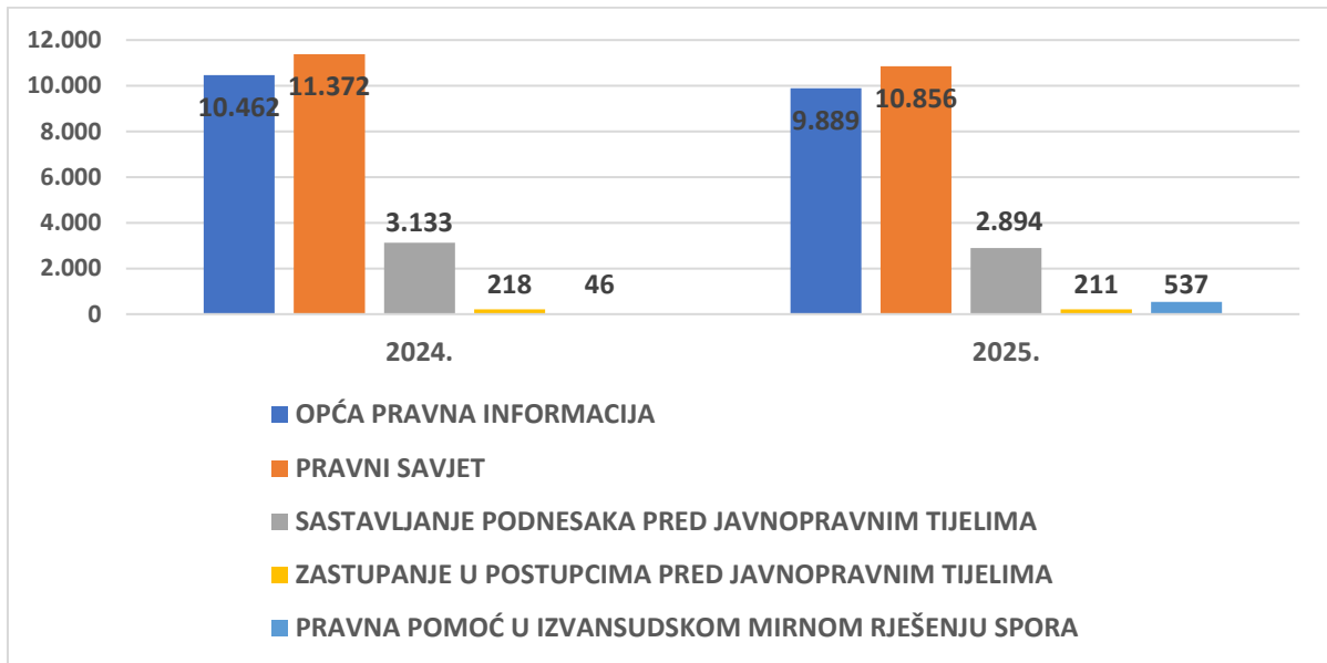
Grafikon 3.
