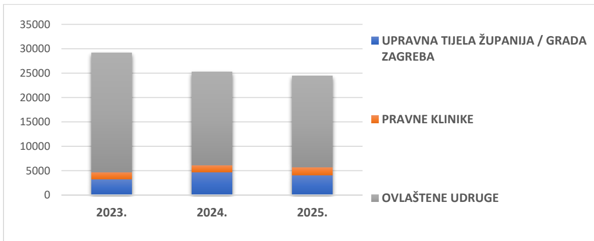
Grafikon 4.
