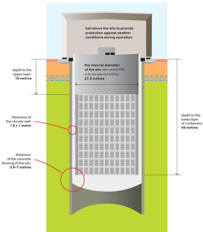
Slika 3-6 Prikaz poprečnog presjeka silosa tijekom rada.
