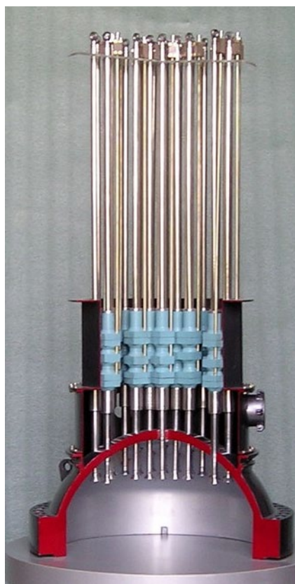
Slika 7-9: Primjeri poklopca RPV-a
